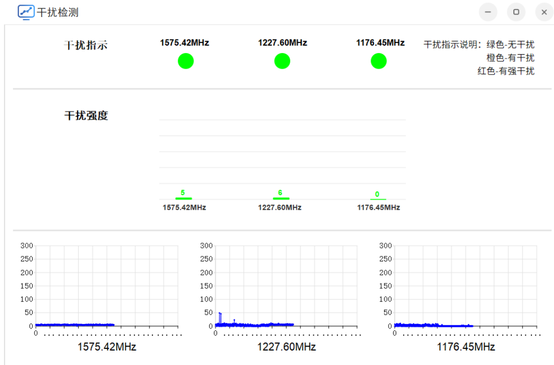
图 3-23 干扰检测
