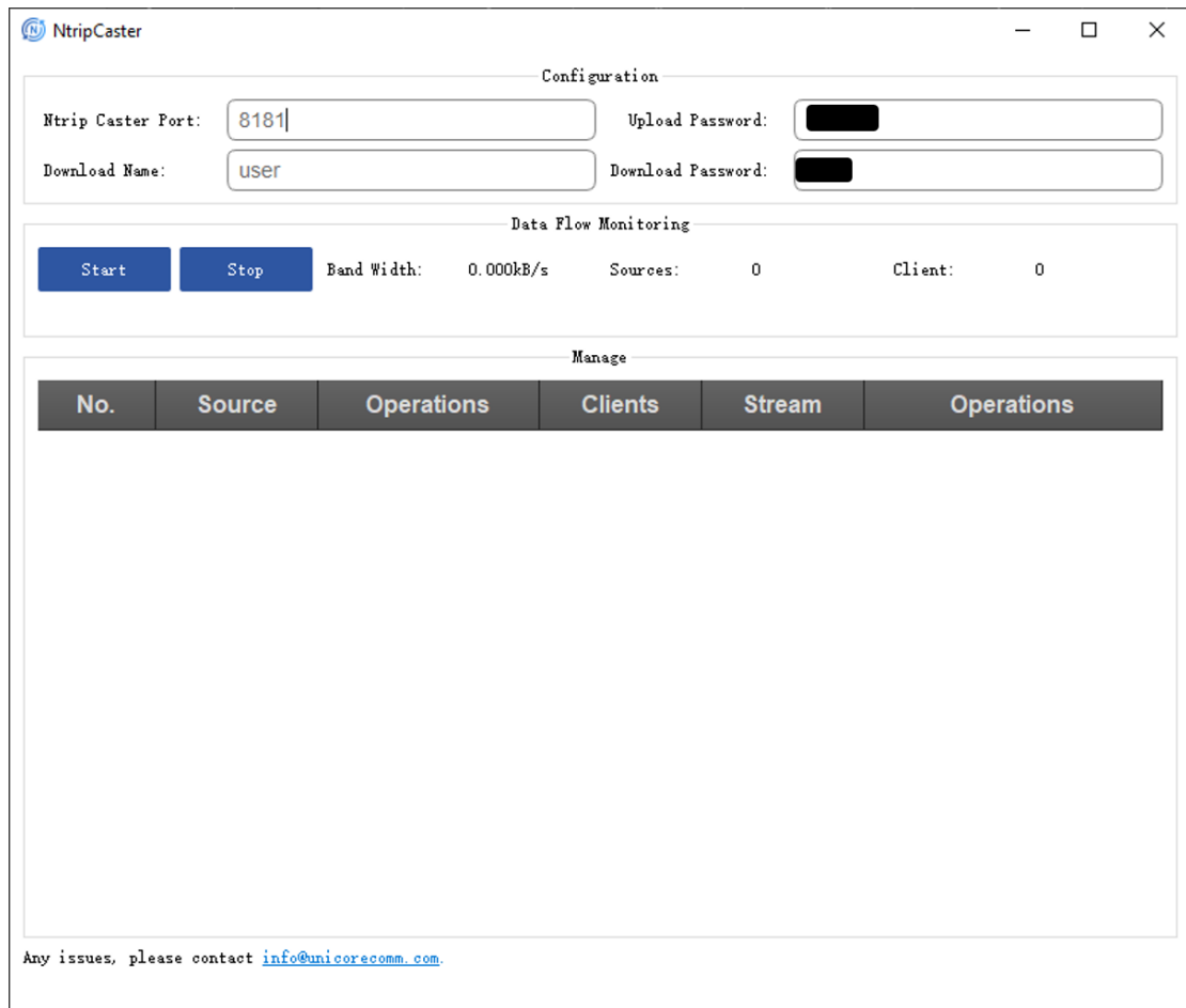
图 3-41 NtripCaster 窗体
