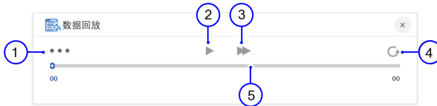
图 3-18 数据回放
