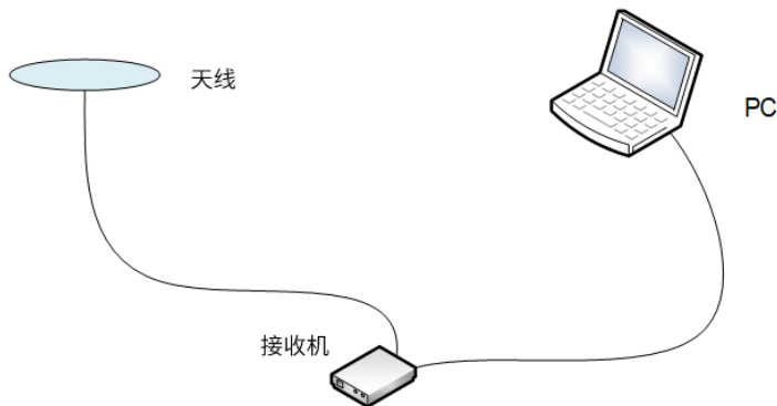
图 3-1 连接示意图
