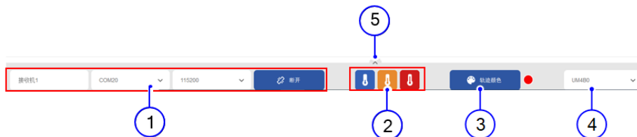
图 2-4 状态栏
