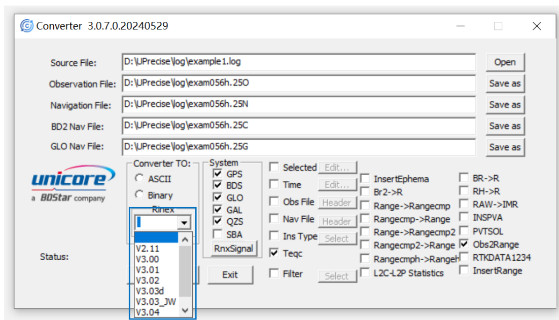
图 3-37 数据转换 (2)
