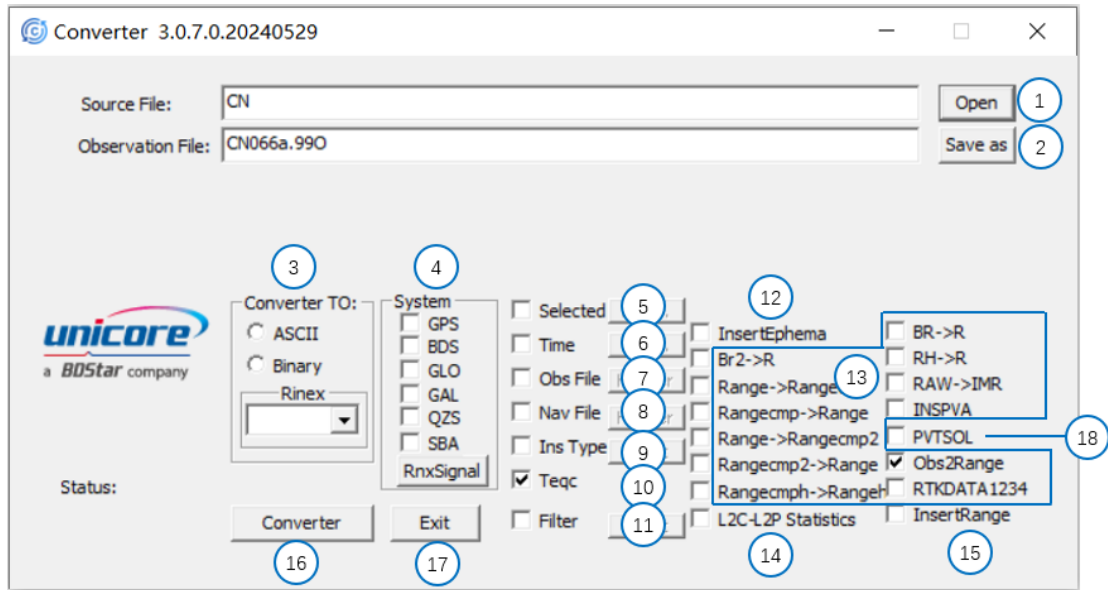
图 3-39 数据转换 (4)
