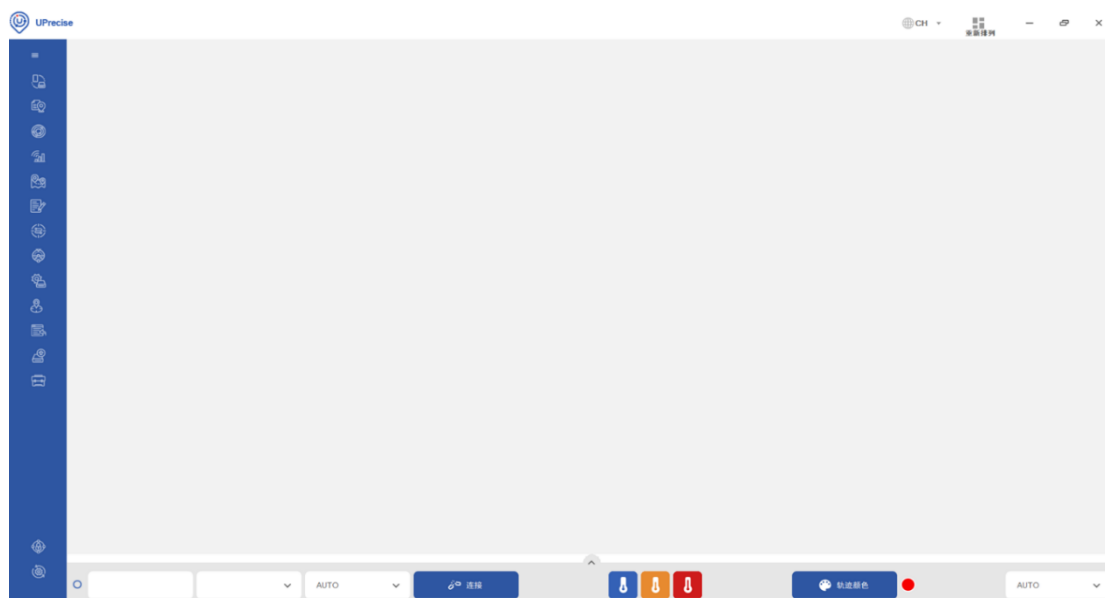
图 1-3 UPrecise 主界面
