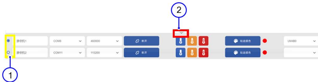
图 2-5 展开效果
