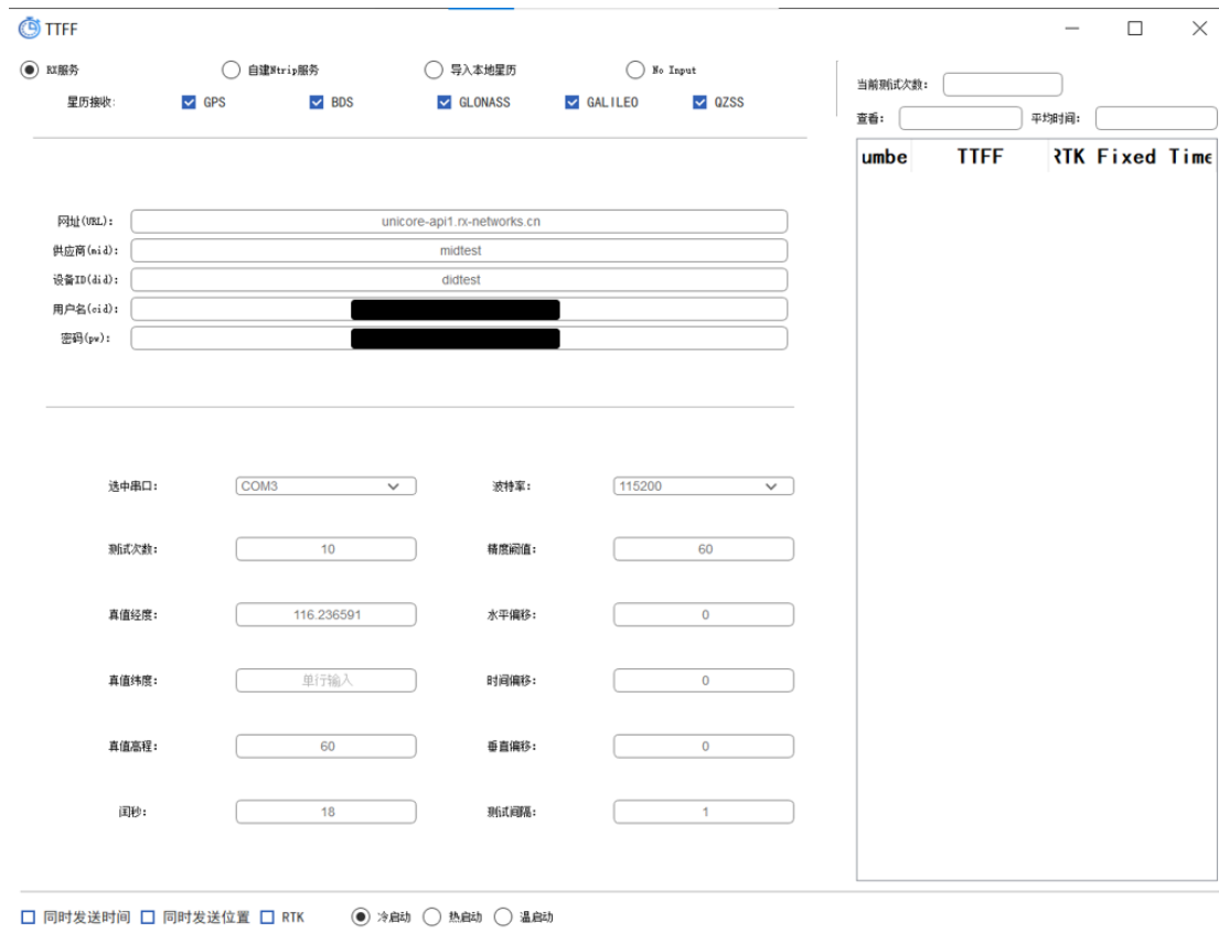
图 3-32 TTFF 窗体
