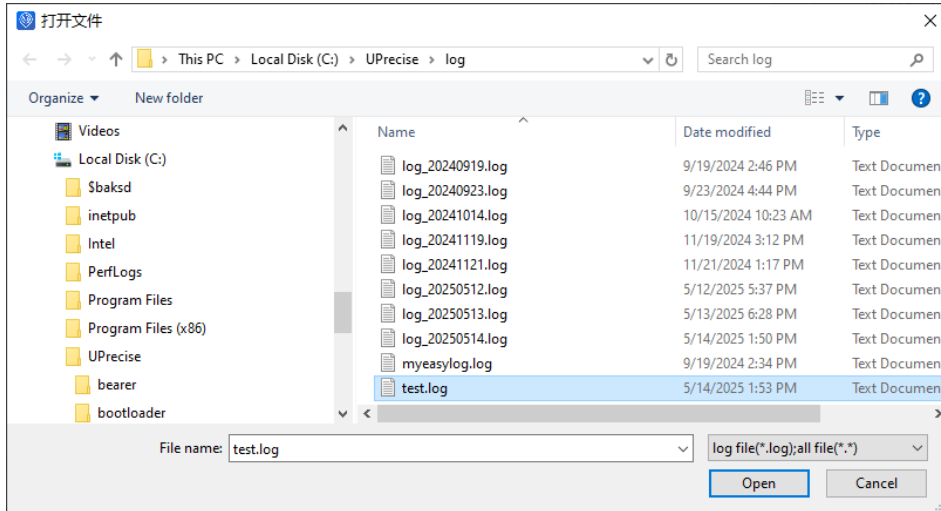
图 3-19 打开文件
