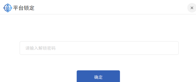
图 3-45 平台解锁
