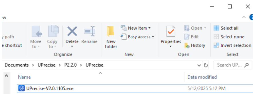
图 1-1 运行安装包
