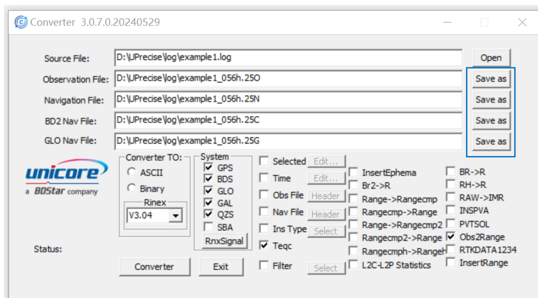
图 3-38 数据转换 (3)
