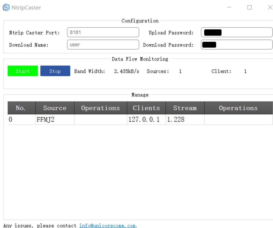
图 3-42 NtripCaster 信息
