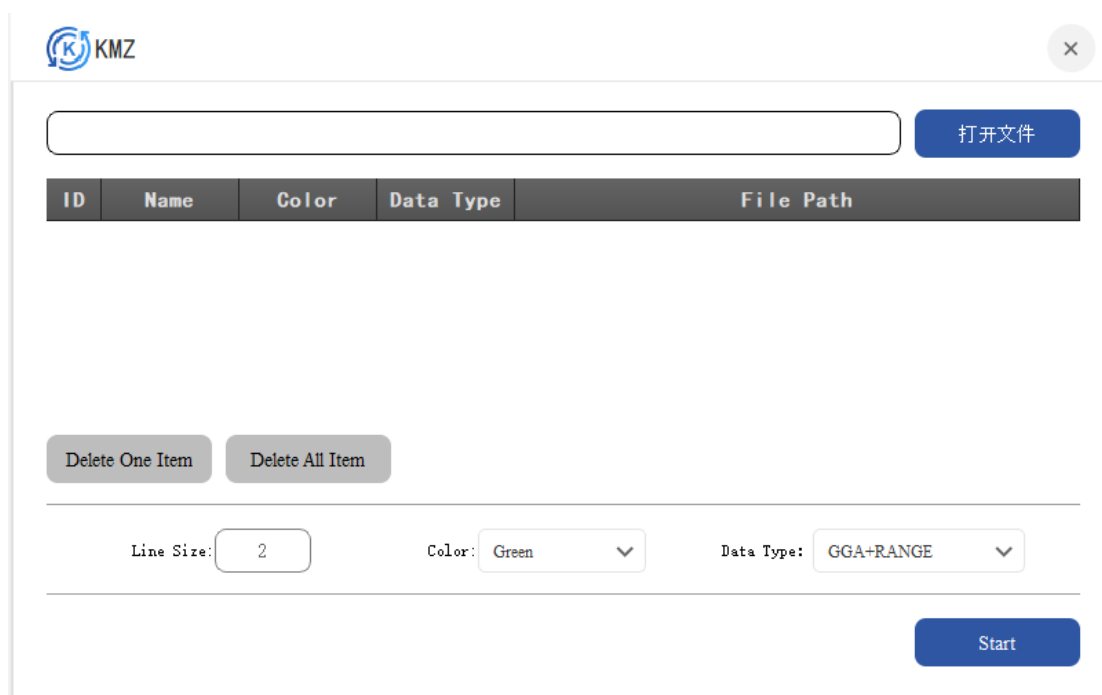
图 3-29 KMZ 窗体
