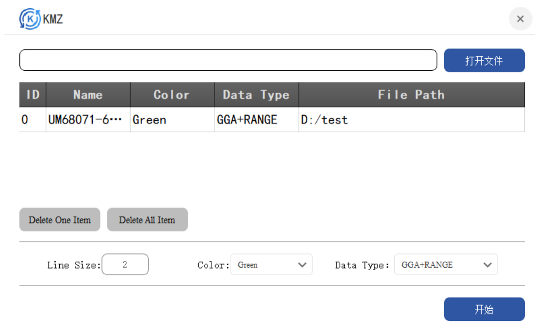
图 3-30 KMZ 文件
