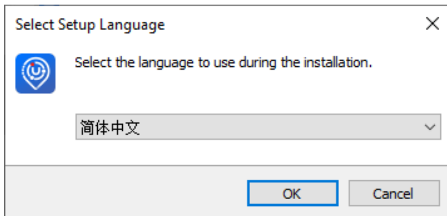
图 1-2 选择语言
