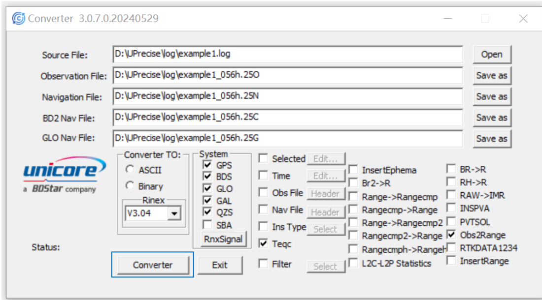
图 3-40 数据转换（5）
