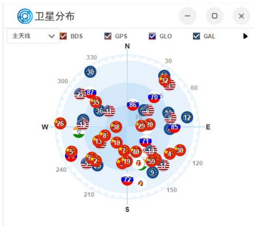
图 3-5 卫星分布
