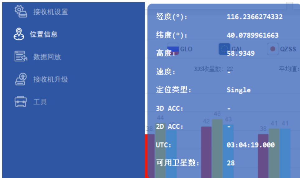
图 3-14 位置信息
