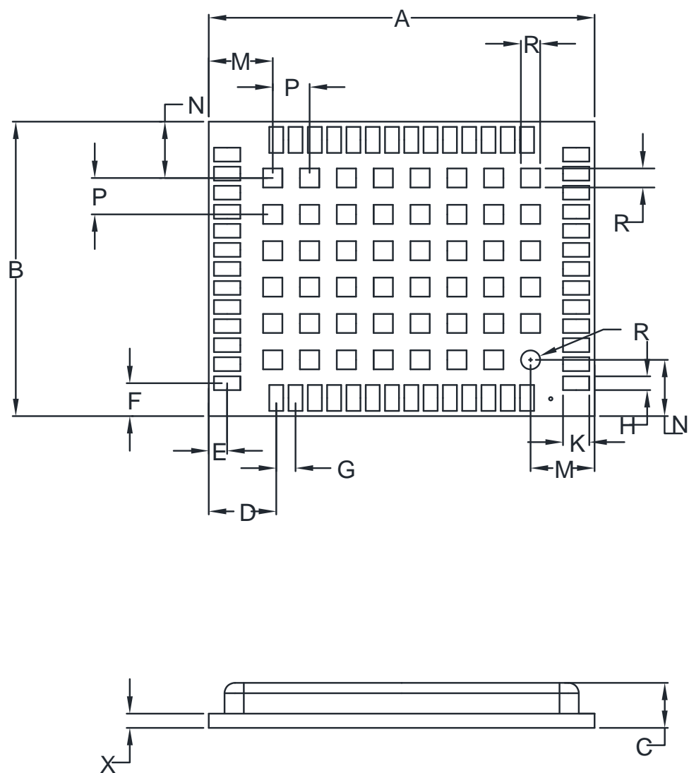
图 3-2 UM681A 机械图
