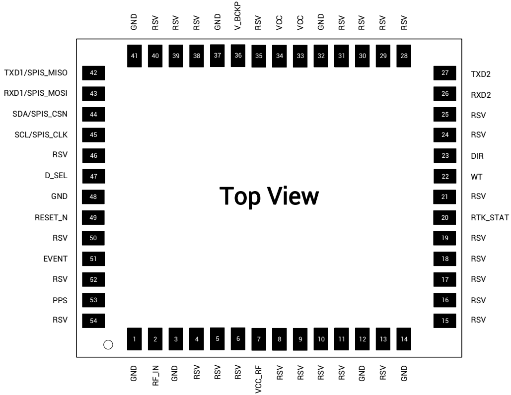
图 3-1 UM681A 管脚图
