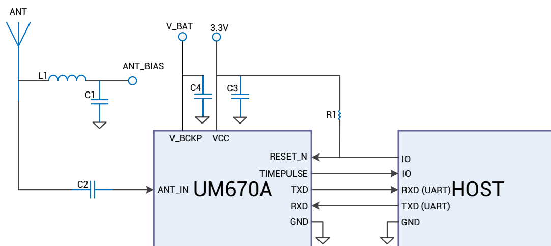
图 3-1 UM670A 最小系统推荐设计
