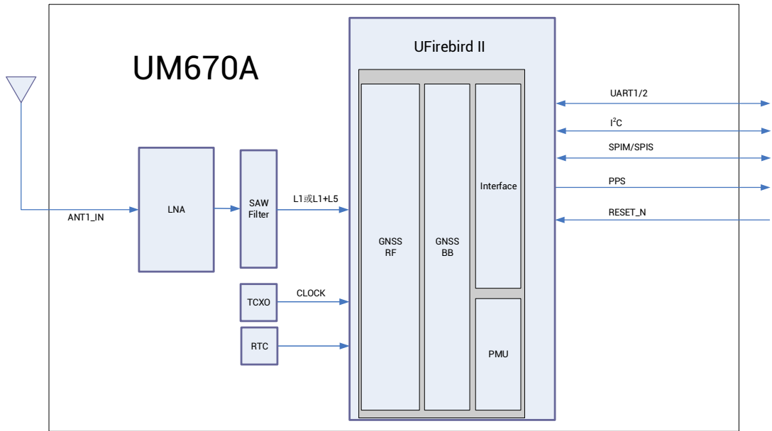
图 1-2 UM670A 结构框图 2
