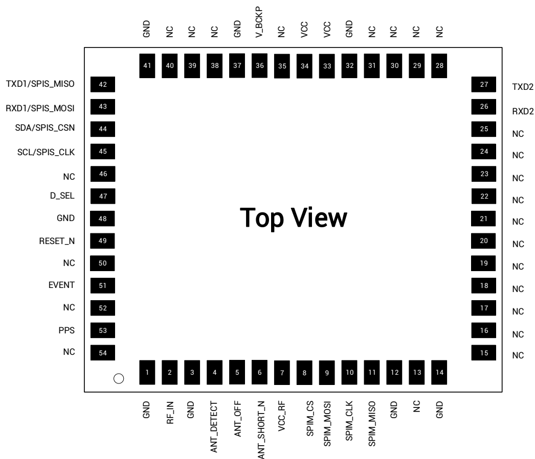
图 2-1 UM670A 管脚图
