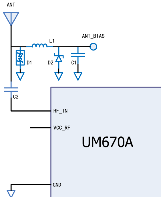
图 3-2 UM670A 外部天线馈电参考电路
