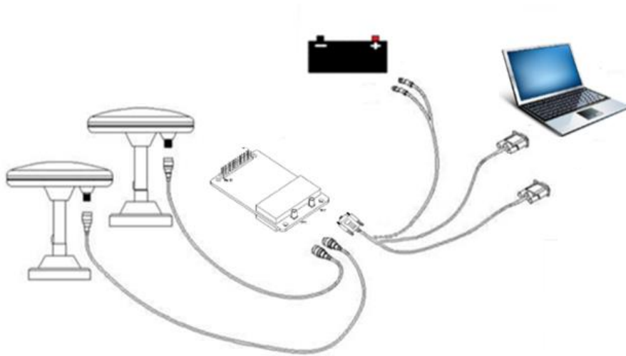
图 4-1 连接示意图
