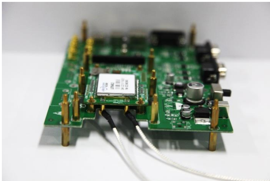
图 4-3 连接天线
