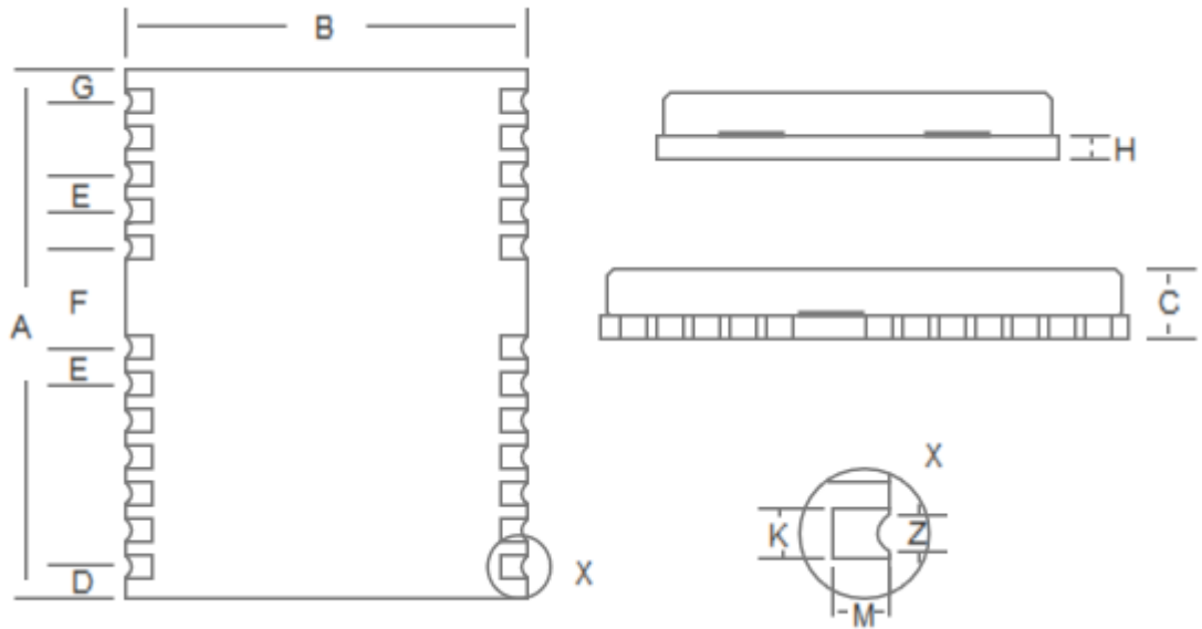
图 3-1 机械图
