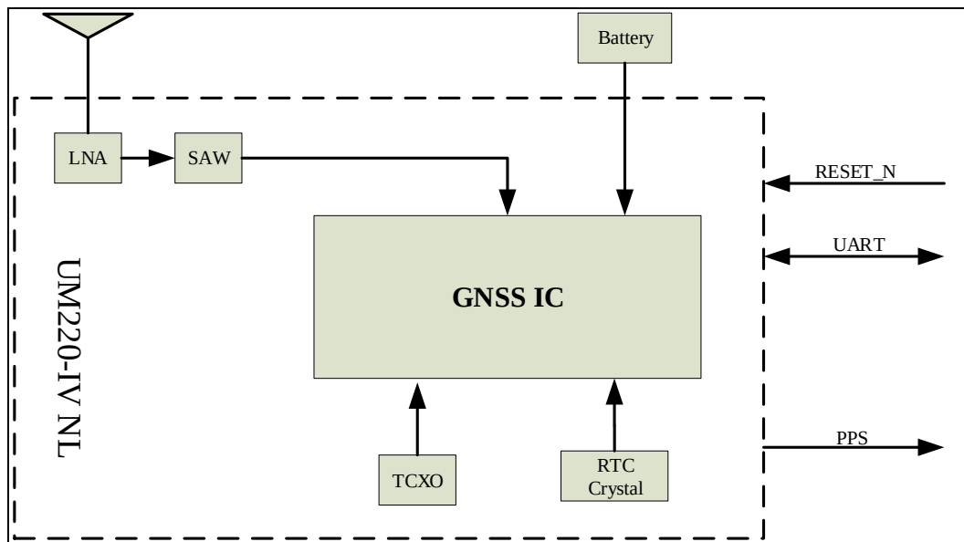
图 1-2 结构框图
