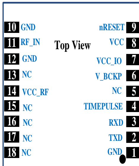
图 3-2 UM220-IV M0 管脚图
