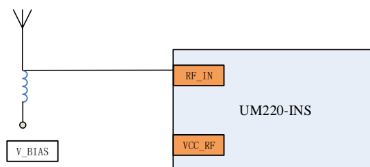
图 4-1 UM220-INS 系列模块的有源天线方案
