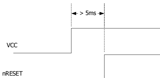
图 4-3 UM220-INS 模块复位信号
