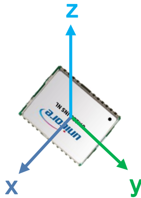
图 4-6 模块坐标系
