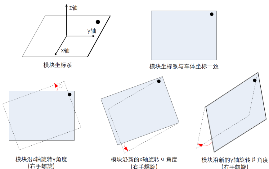
图 4-8 模块旋转示意图
