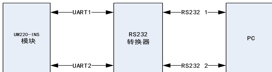
图 4-4 串口连接到 PC
