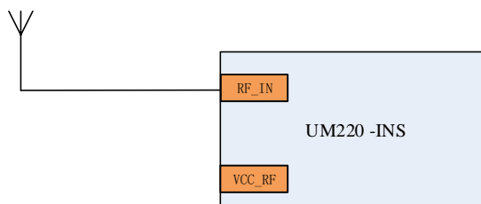
图 4-2 UM220-INS 系列模块无源天线方案
