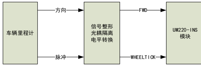
图 4-5 里程计的连接
