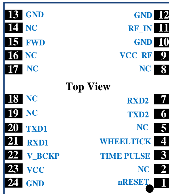
图 3-2 管脚图
