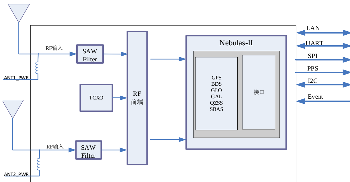
图 1-2 UB482 结构框图
