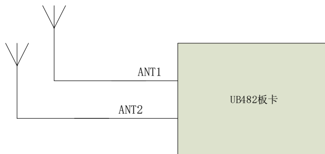
图 3-2 UB482 天线连接示意图
